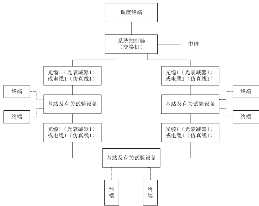
图2 环形系统设备连接
