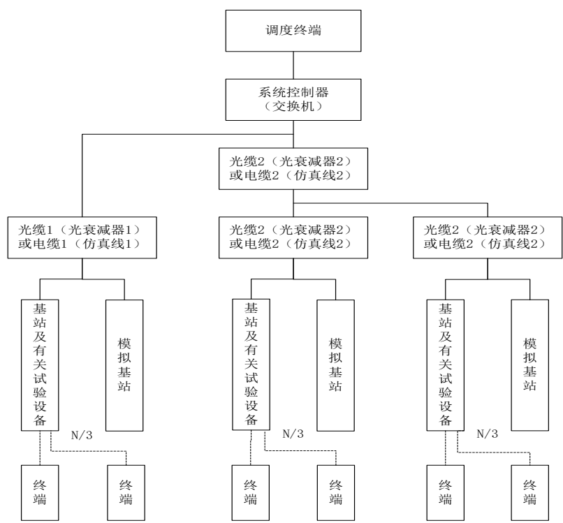
图1 树形系统设备连接
