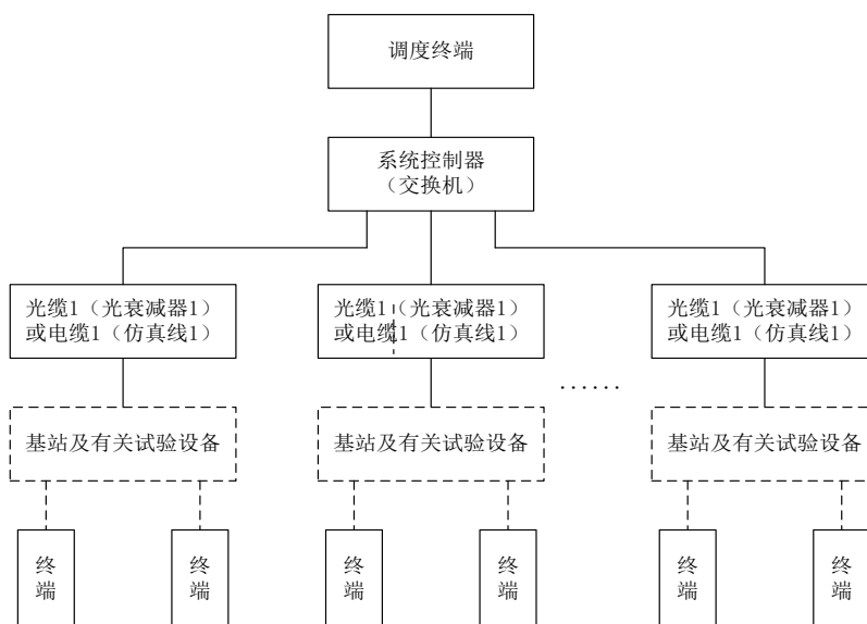
图3 星形系统总线型系统设备连接
