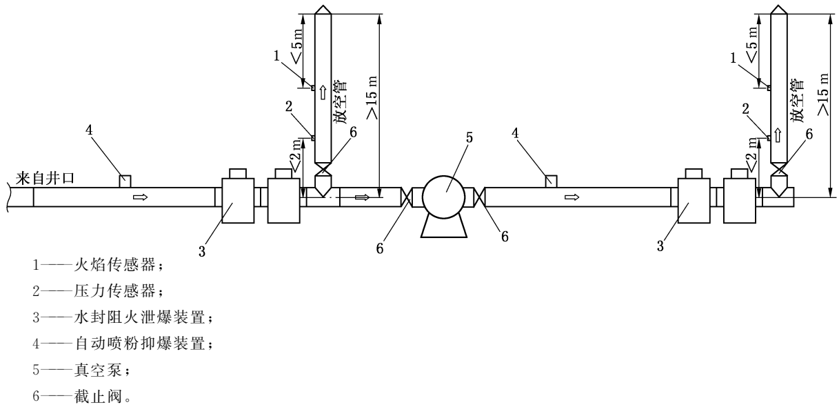
图 2 地面瓦斯排空系统安全设施安装示意图
